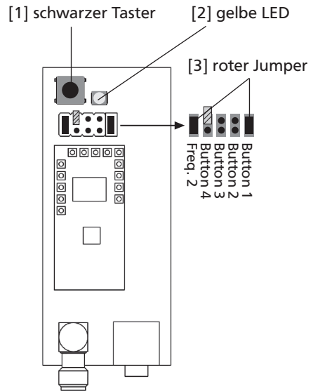
Abb. 4: Frequenz 2 gewählt und Taste 1 als Auslösetaste aktiviert, der Jumper auf Button 4 ist inaktiv.
