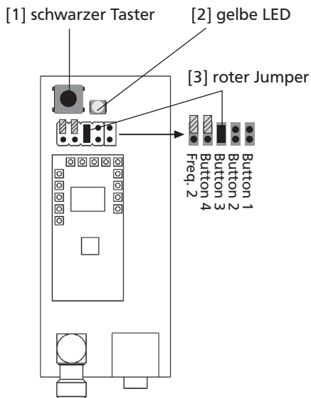
Abb. 2: Taste 3 als Auslösetaste aktiviert, die Jumper auf Button 4 und Freq. 2 sind inaktiv.
