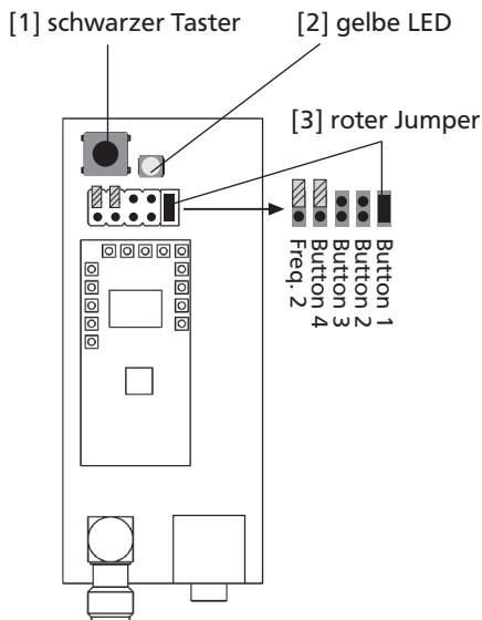
Abb. 1: Taste 1 als Auslösetaste aktiviert, die Jumper auf Button 4 und Freq. 2 sind inaktiv.
