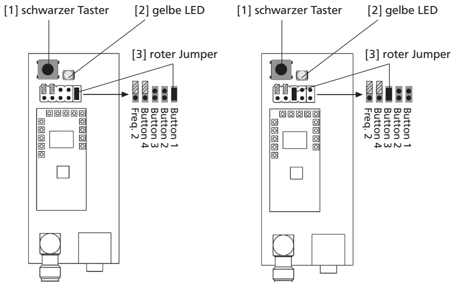
Abb. 1: Taste 1 als Auslösetaste aktiviert, die Jumper auf Button 4 und Freq. 2 sind inaktiv.
